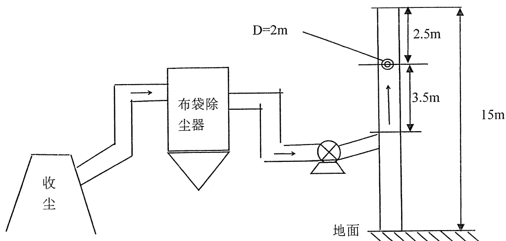
图 4-1 2#、3#原煤破碎合用除尘器监测点位示意图
