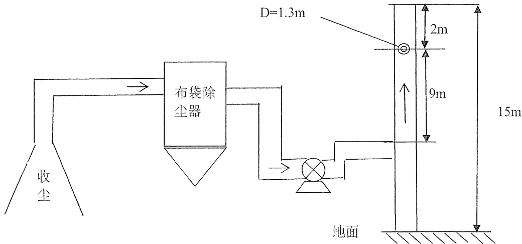
图 4-1 60 万吨精煤破碎监测点位示意图
