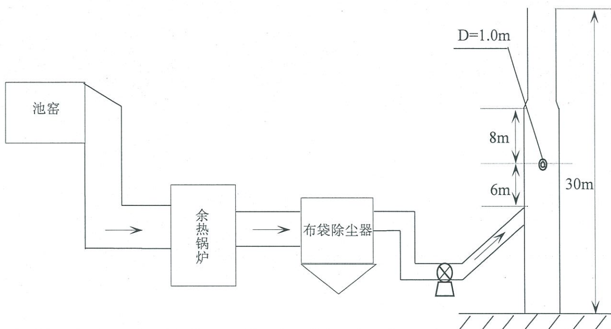
图 4-1 池窑烟气袋式除尘器出口示意图
