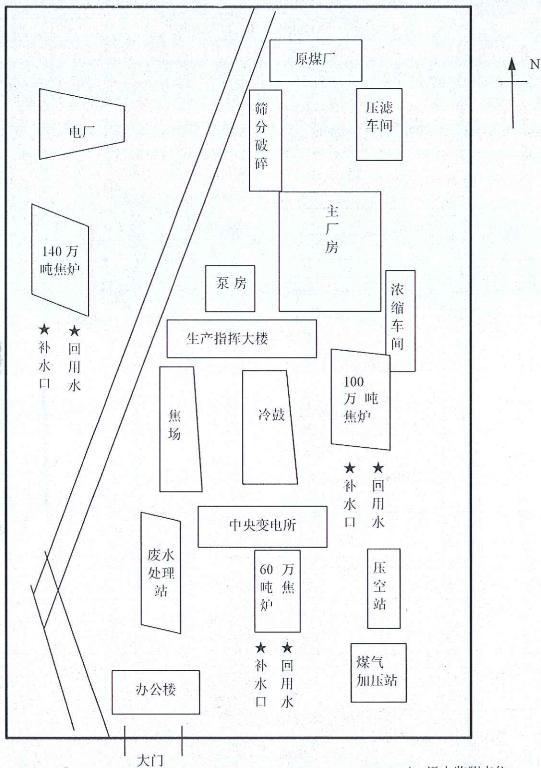
图 4-1 污水监测点位平面示意图
