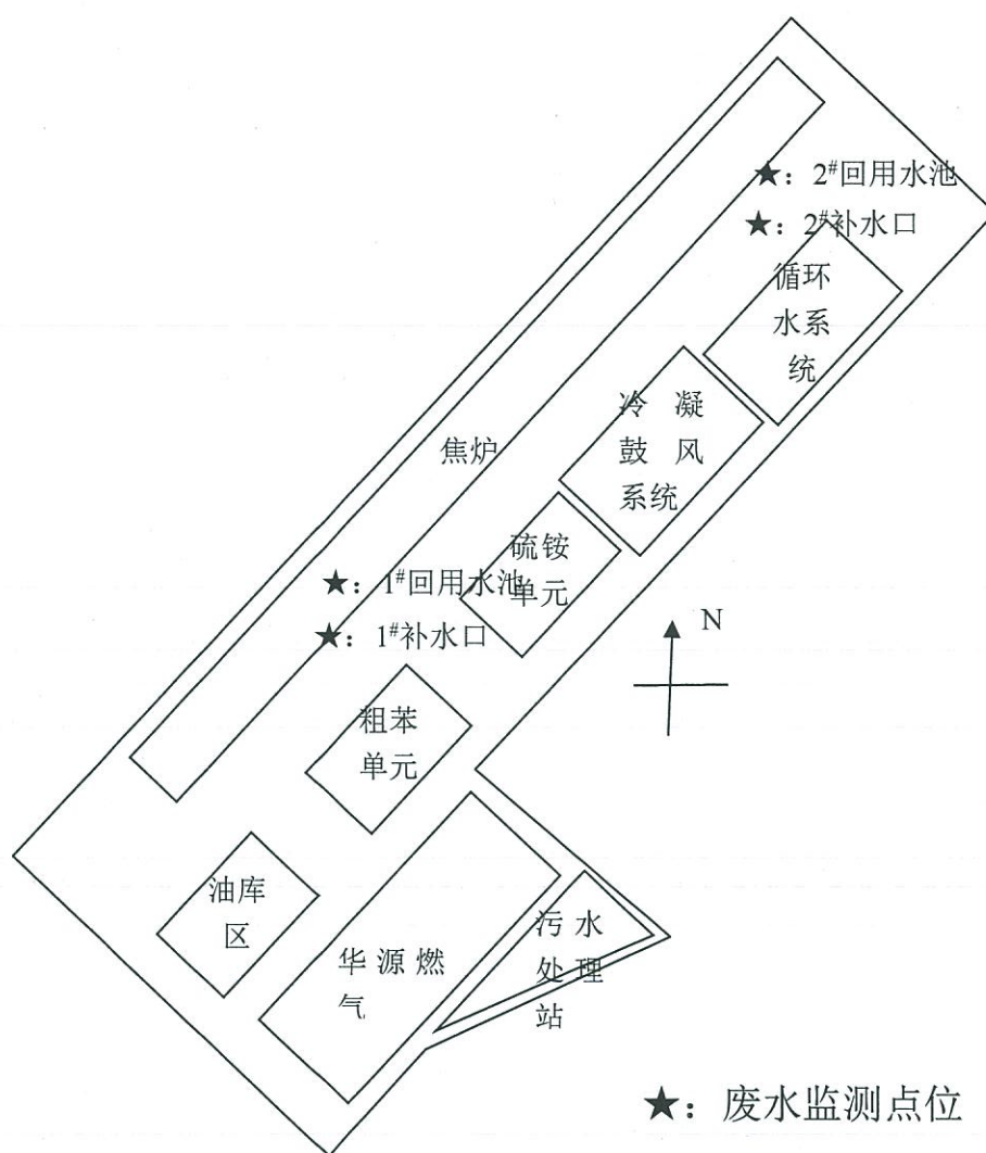
图 4-1 湿熄焦水池监测点位平面示意图
