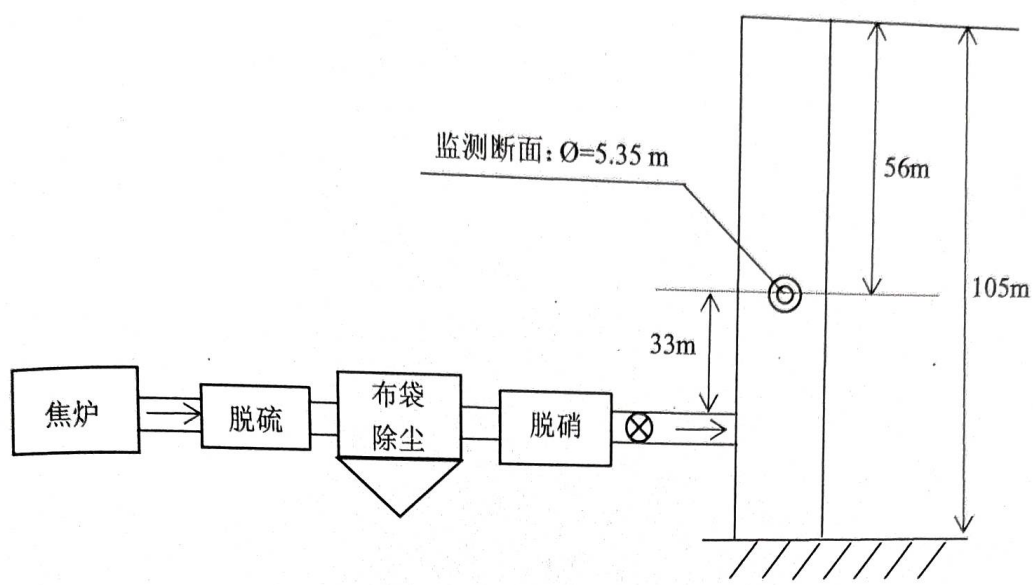
图 5-1 140 万吨 5# 烟囱有组织废气监测点位示意图
